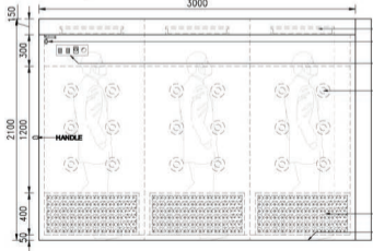
ELEVATION-A SCALE 1:35
